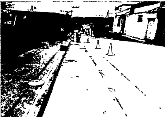
Trazo y corte de disco en pavimento hidráulico
