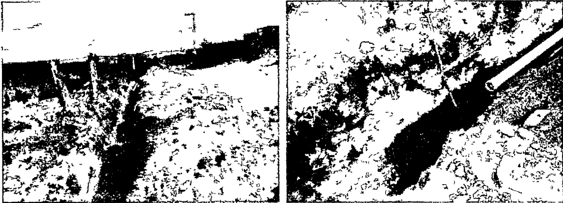
Plantilla apisonada al 85% proctor en zanjas con material producto de banco.
