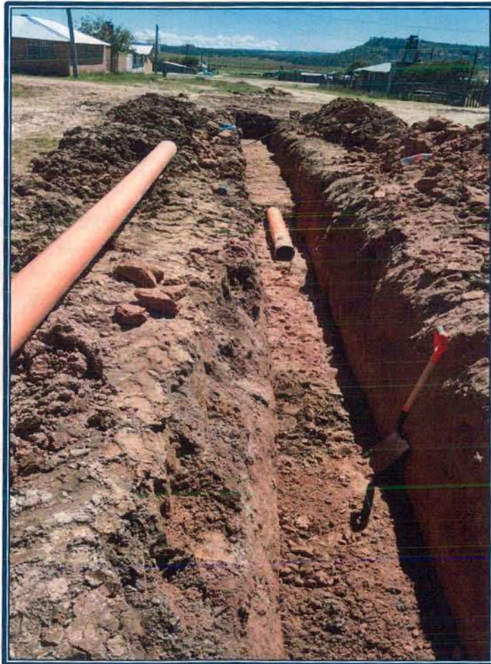
SISTEMA DE ALCANTARILLADO, RED DE ATARJEAS Y DESCARGAS DOMICILIARIAS POB. BANDERAS DEL ÁGUILA
