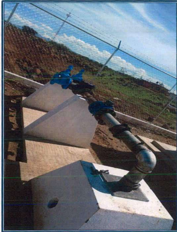
SISTEMA DE AGUA POTABLE, EQUIPAMIENTO DE POZO PROFUNDO, DESCARGA HIDRÁULICA, LÍNEA DE CONDUCCIÓN, CERCO DE PROTECCIÓN, ELECTRIFICACIÓN, CASETA DE CLORACIÓN
