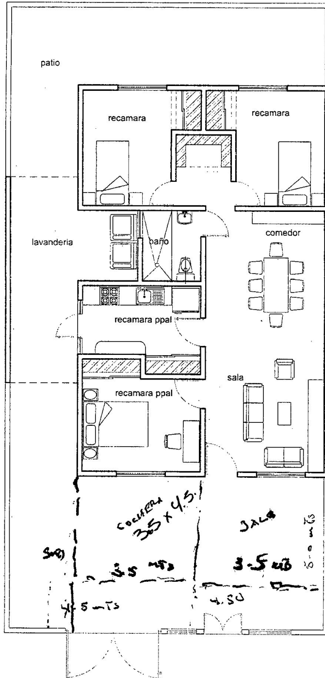
PLANTA ESTADO ACTUAL
