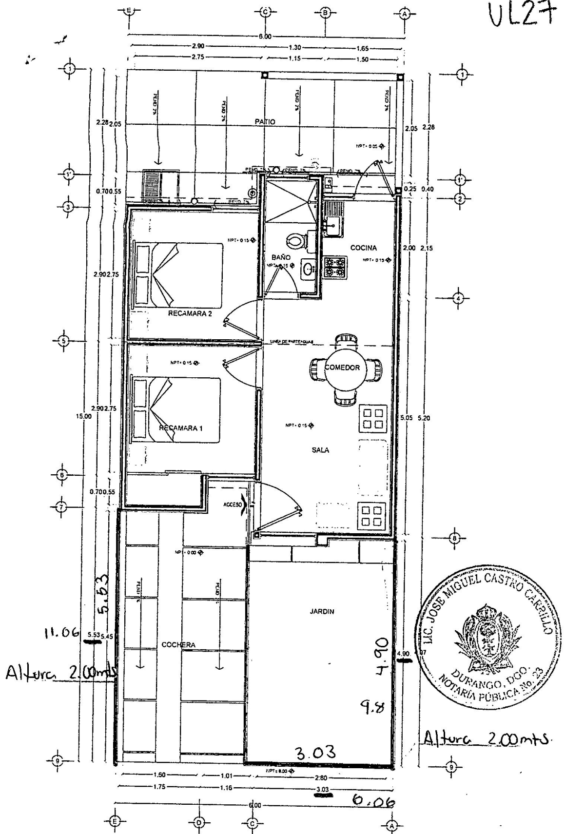
PLANTA ARQUITECTÓNICA 42.90 m 2
