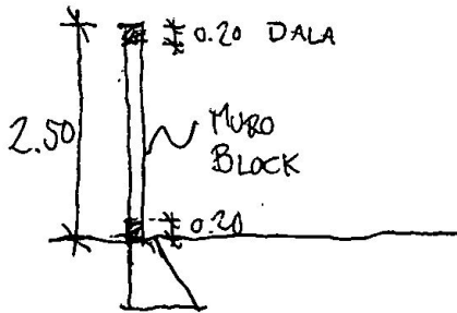
SECCION (VISTA CORTE)
