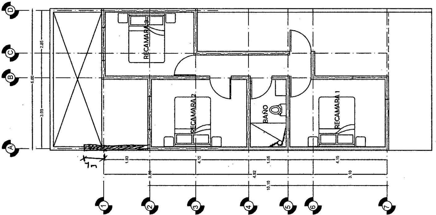
PLANTA
