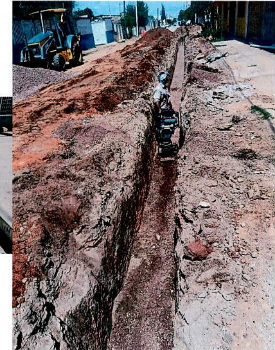
AGUA POTABLE EN CALLE IGNACIO LÓPEZ TARSO, ENTRE ELEAZAR GARÍA Y PEDRO INFANTE COL. VALLE DEL GUADIANA
