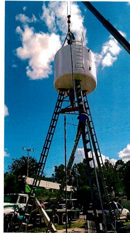
REHABILITACIÓN DE TANQUE DE ALMACENAMIENTO - POB. SAN JOSÉ DEL MOLINO
