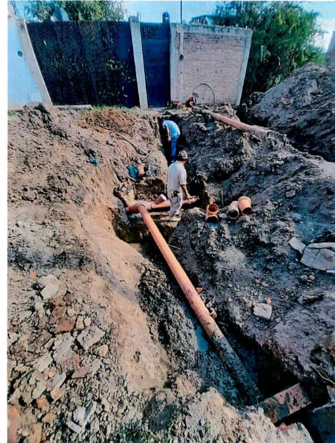
DESCARGAS DOMICILIARIAS EN CALLE BEGONIA COL. VALLE DEL SUR
