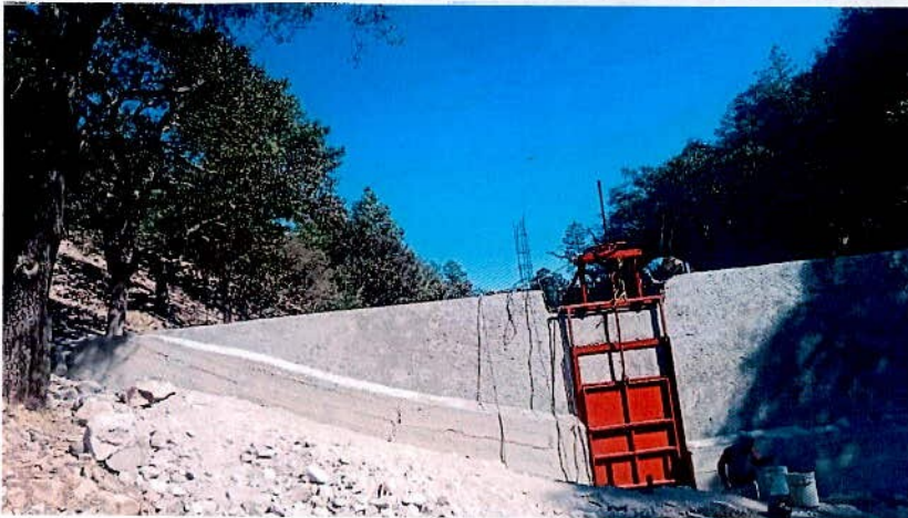
REHABILITACIÓN DE PRESA DE MAMPOSTERIA POB. MESAS DE URBINA
