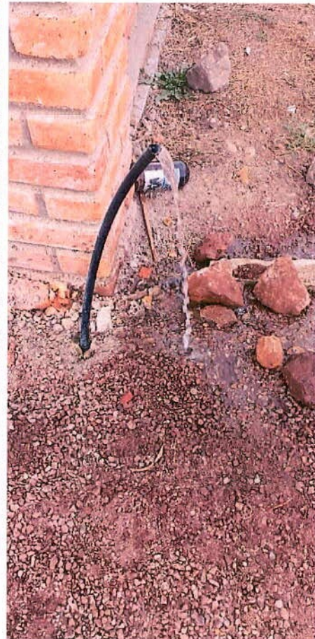
CONSTRUCCIÓN DE LÍNEA CONDUCCIÓN - POB. CINCO DE FEBRERO
