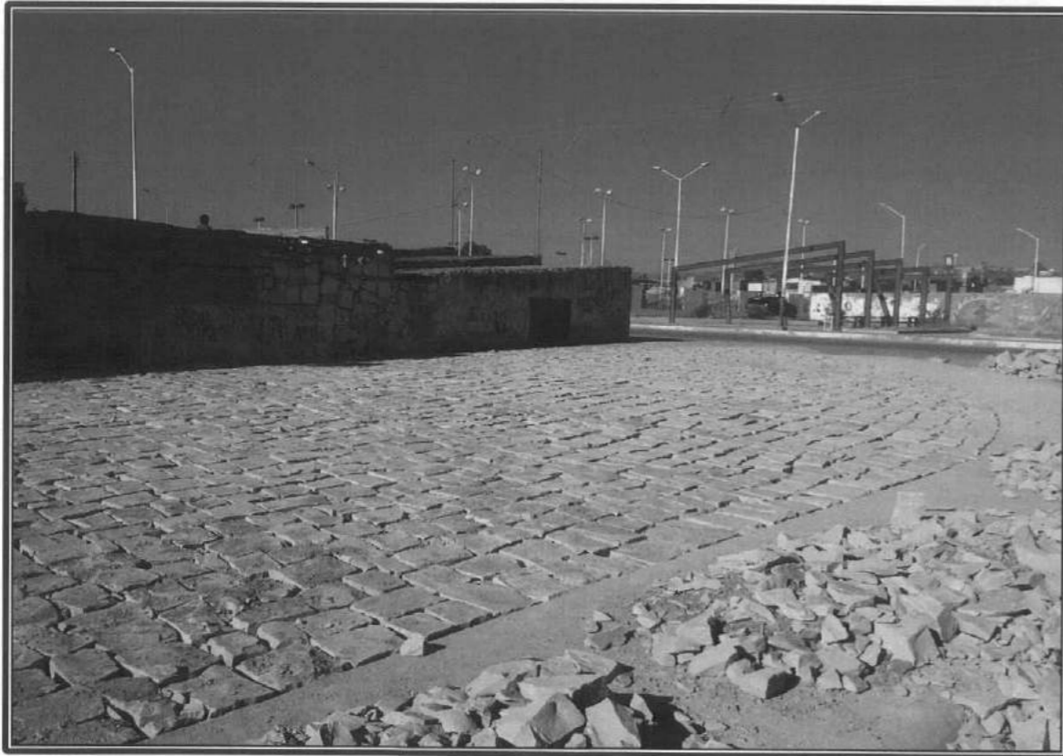
CONSTRUCCIÓN DE LA VIALIDAD LAS MANGAS (Ia. ETAPA) VICTORIA DE DURANGO
