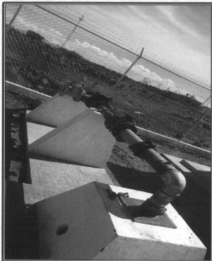
SISTEMA DE AGUA POTABLE, EQUIPAMIENTO DE POZO PROFUNDO, DESCARGA HIDRÁULICA, LÍNEA DE CONDUCCIÓN, CERCO DE PROTECCIÓN, ELECTRIFICACIÓN, CASETA DE CLORACIÓN
