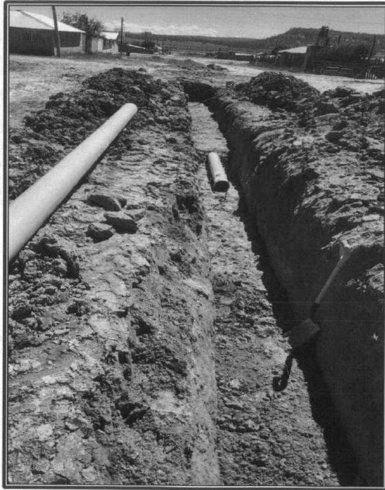
SISTEMA DE ALCANTARILLADO, RED DE ATARJEAS Y DESCARGAS DOMICILIARIAS POB. BANDERAS DEL ÁGUILA
