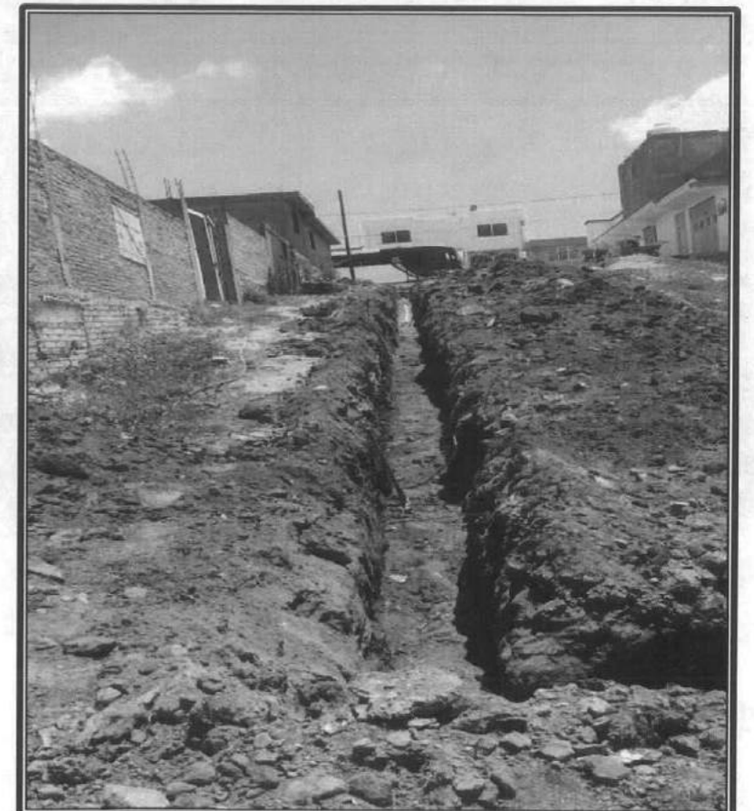
RED DE AGUA POTABLE COL. VALENTÍN GÓMEZ FARÍAS
